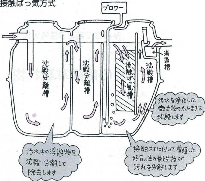
分離接触ばっ気方式
