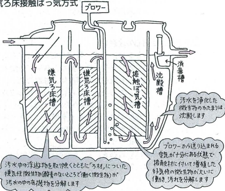
嫌気ろ床接触ばっ気方式
