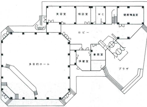
1階平面図
