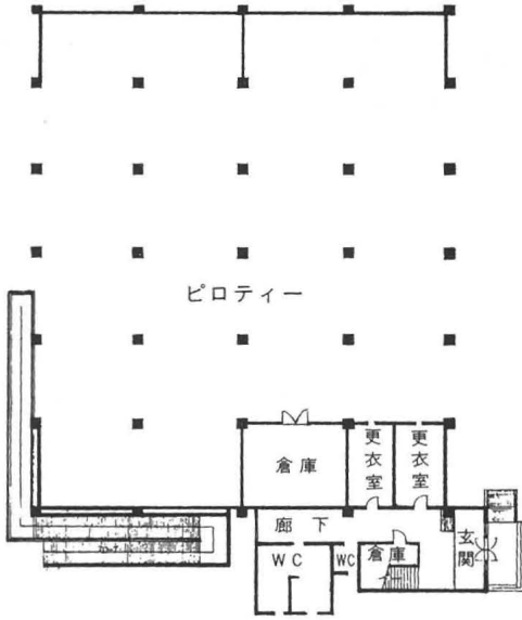
3階平面図
