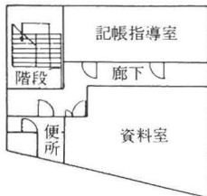
3階平面図
