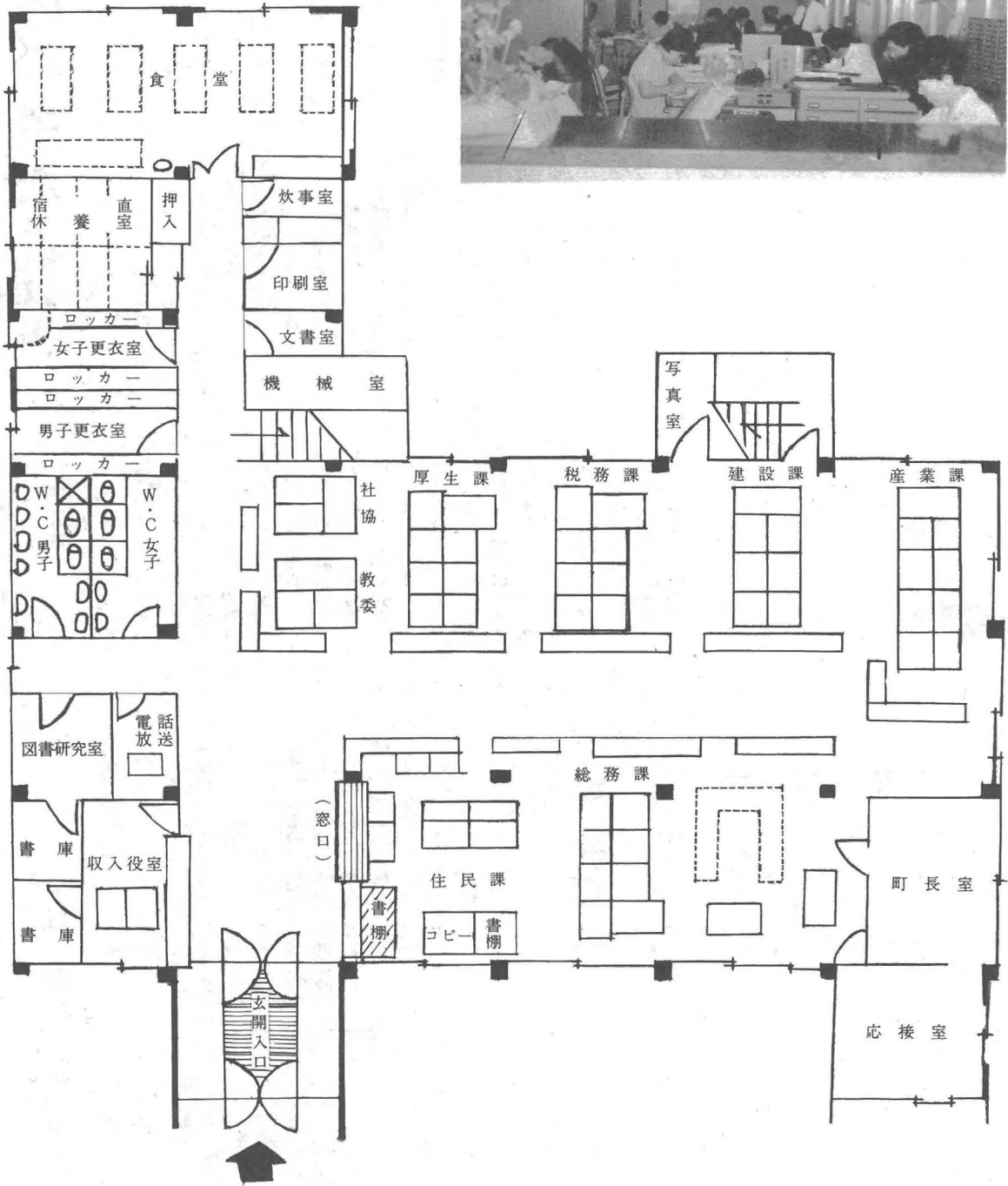
勝浦町役場一階見取図
