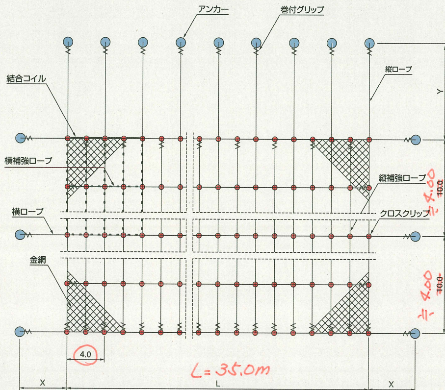
覆式ロックネット 構造図
