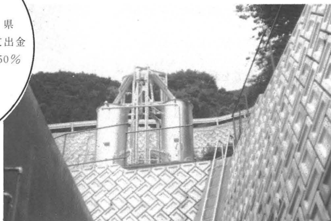
→完成した急速ろ過器
