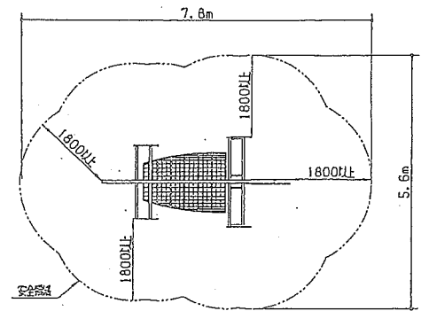
安全柵 平面図 1/100
