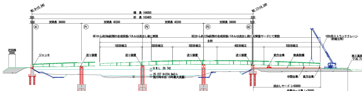
側面図
