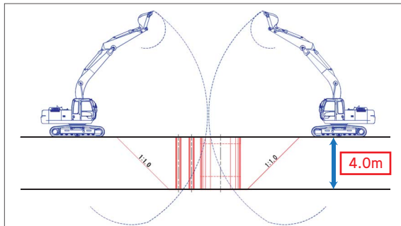
図 開削撤去工法による基礎工撤去
