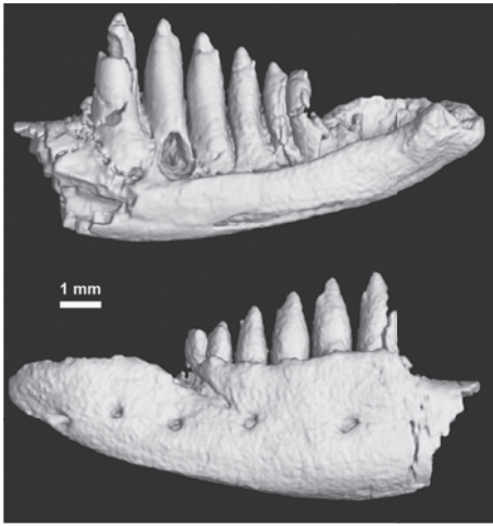
3次元再構築モデル （上：内側、下：外側）
