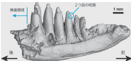
発見されたトカゲ類化石の特徴 （内側から見た図）
