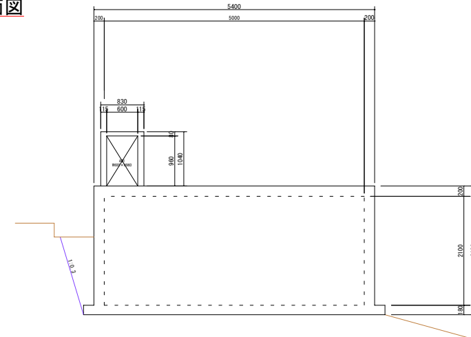
立面図
