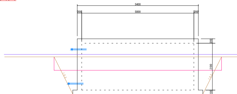
A-A立面図
