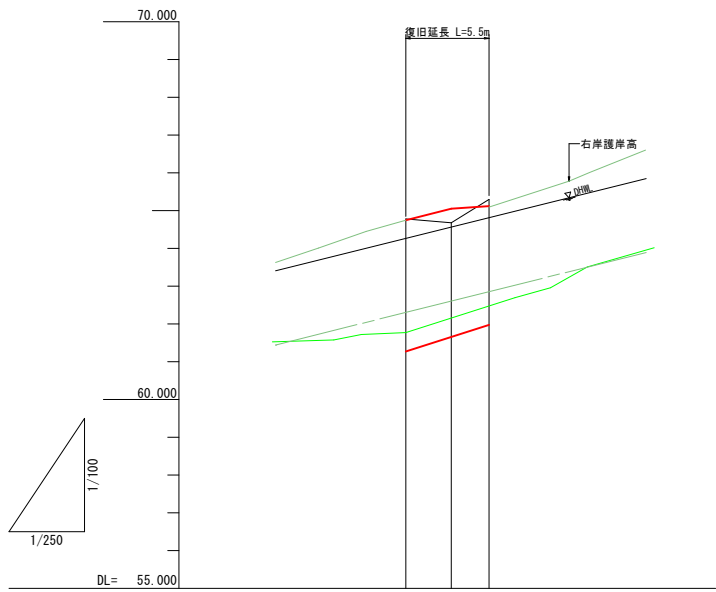
縦断面図
