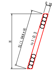
すりつけ工（練石積） S=1/50
