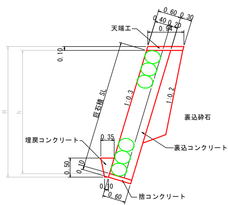
巨石積断面図 S=1/50
