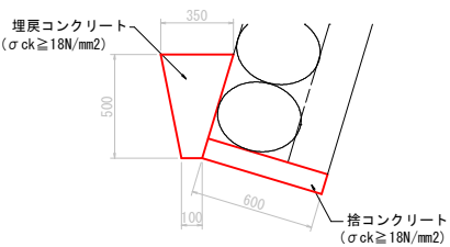
埋戻コンクリート 捨コンクリート S=1/20
