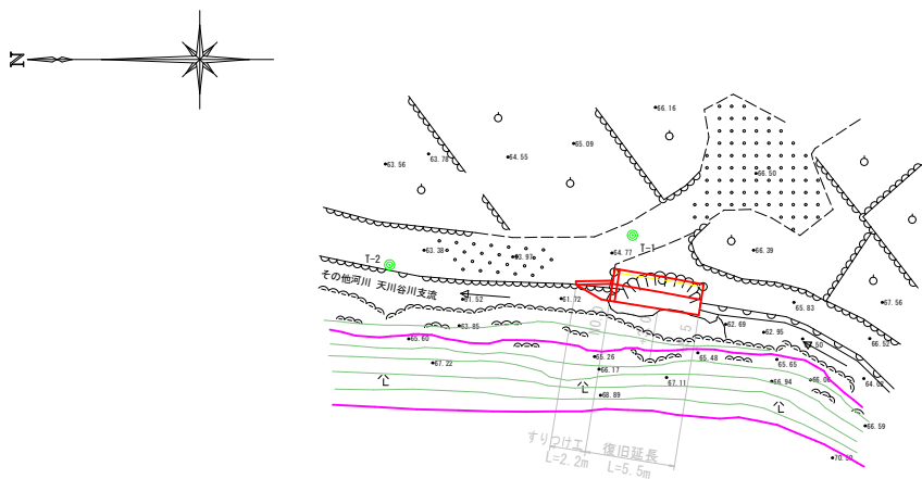
平面図 S=1/250
