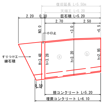
巨石積断面図 S=1/50
