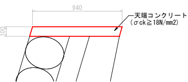
天 端 工 S=1/20
