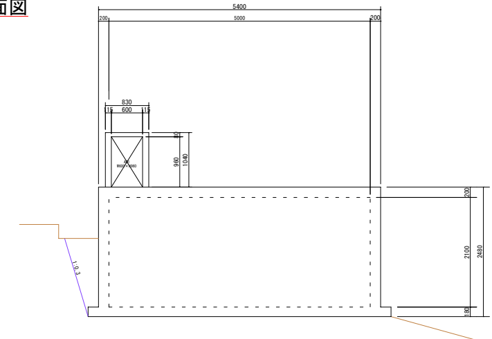
立面図
