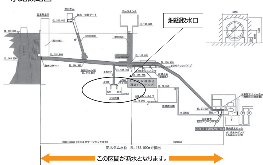
水路概略図 (延長 約6km)
